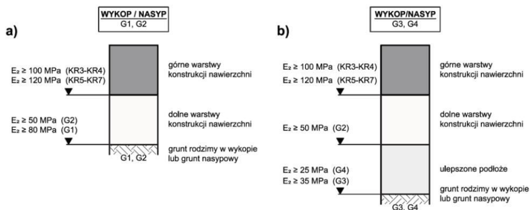
Rys. 3 Schemat układu warstw konstrukcji nawierzchni dla kategorii ruchu KR3-KR7 w wykopie i w nasypie oraz wymagane wartości wtórnych modułów odkształcenia na powierzchni warstw; a) w przypadku grupy nośności podłoża G1 i G2, b) w przypadku grupy nośności podłoża G3 i G4
