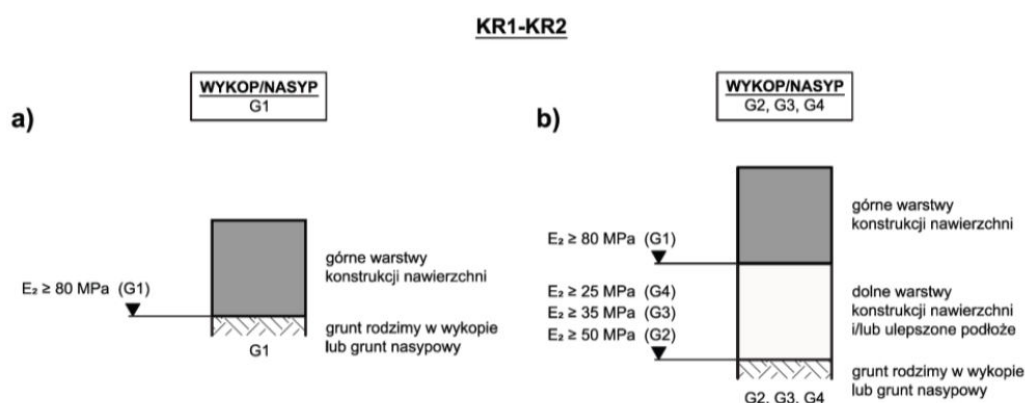
Rys. 2 Schemat układu warstw konstrukcji nawierzchni dla kategorii ruchu KR1-KR2 w wykopie i w nasypie oraz wymagane wartości wtórnych modułów odkształcenia na powierzchni warstw; a) w przypadku grupy nośności podłoża G1, b) w przypadku grupy nośności podłoża G2, G3 i G4
