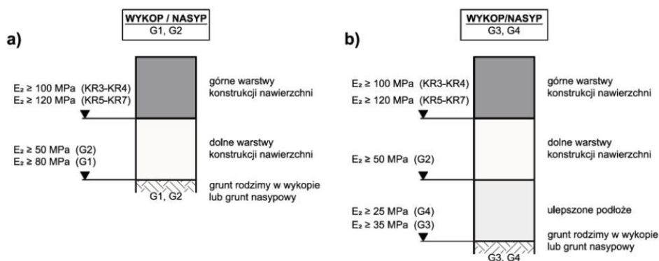
Rys. 3 Schemat układu warstw konstrukcji nawierzchni dla kategorii ruchu KR3-KR7 w wykopie i w nasypie oraz wymagane wartości wtórnych modułów odkształcenia na powierzchni warstw; a) w przypadku grupy nośności podłoża G1 i G2, b) w przypadku grupy nośności podłoża G3 i G4
